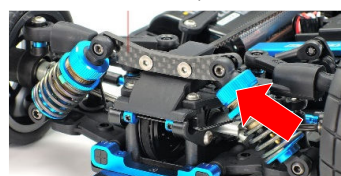
▲ リヤ装着例
