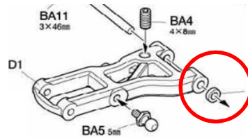
使用例(サスアーム前後位置調整)
